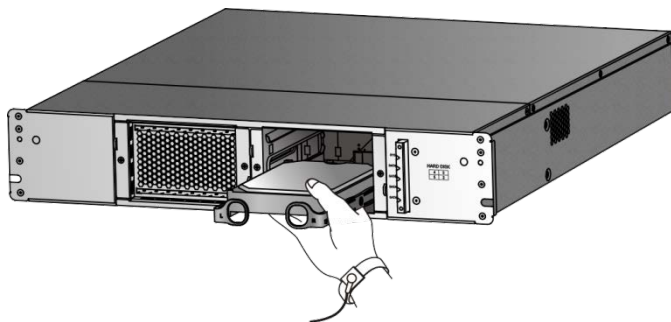
图2-7 插入硬盘
