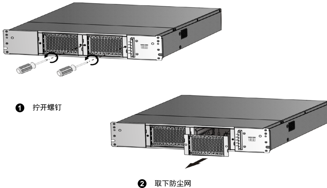
图2-6 拆卸防尘网
