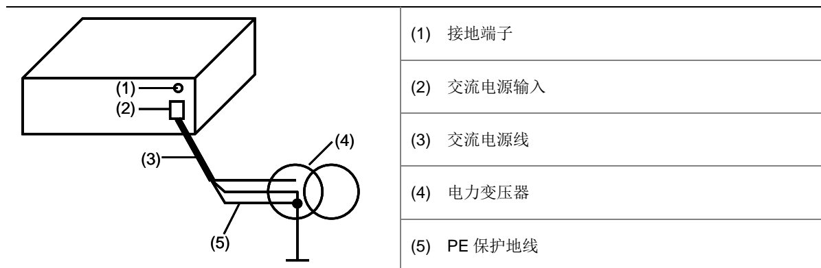
图2-14 接地安装示意图（利用交流 PE 线接地）
