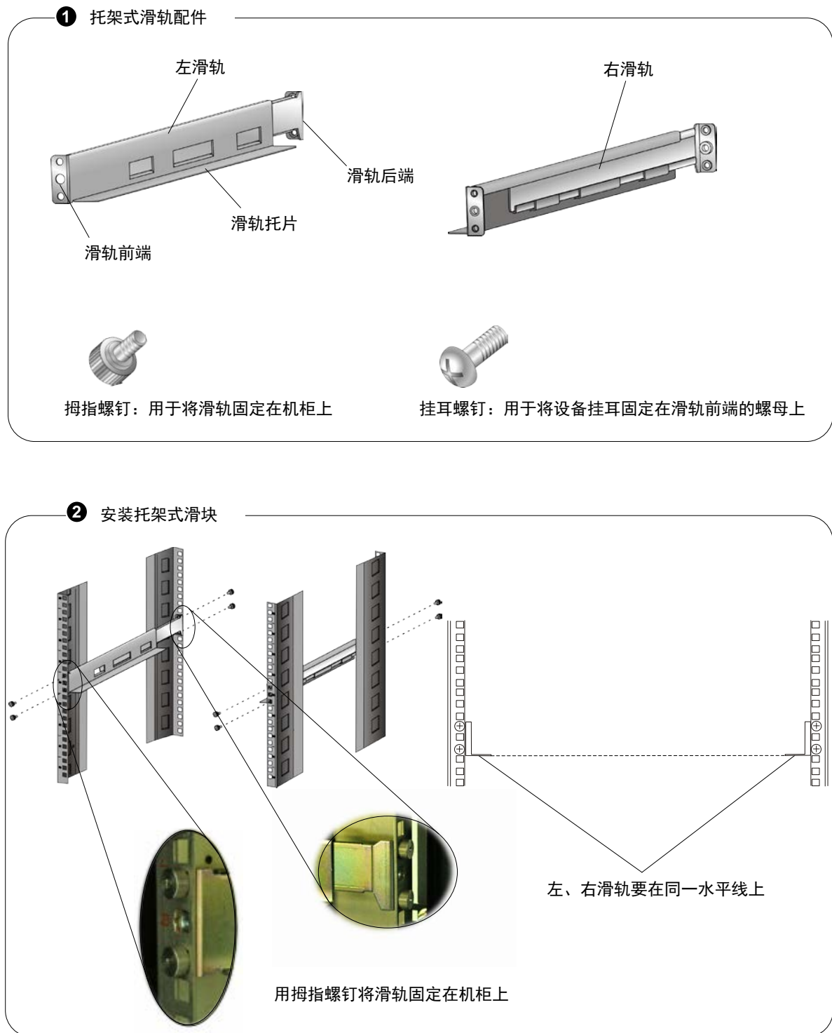
图2-4 安装托架式滑轨
