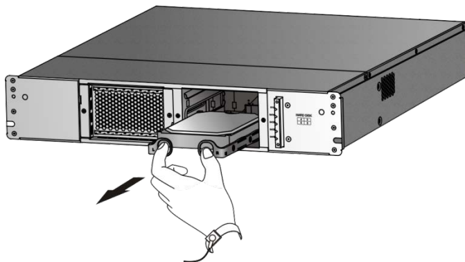
图6-1 拔出硬盘
