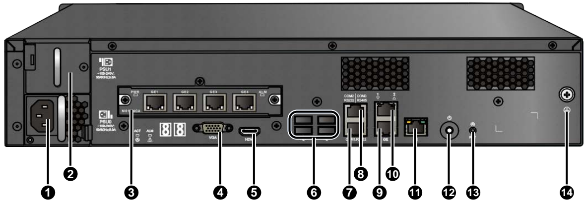
图1-3 后面板接口/按钮
