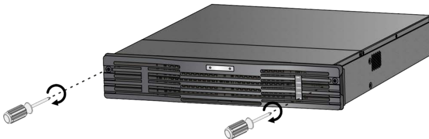
图2-9 安装前面板
