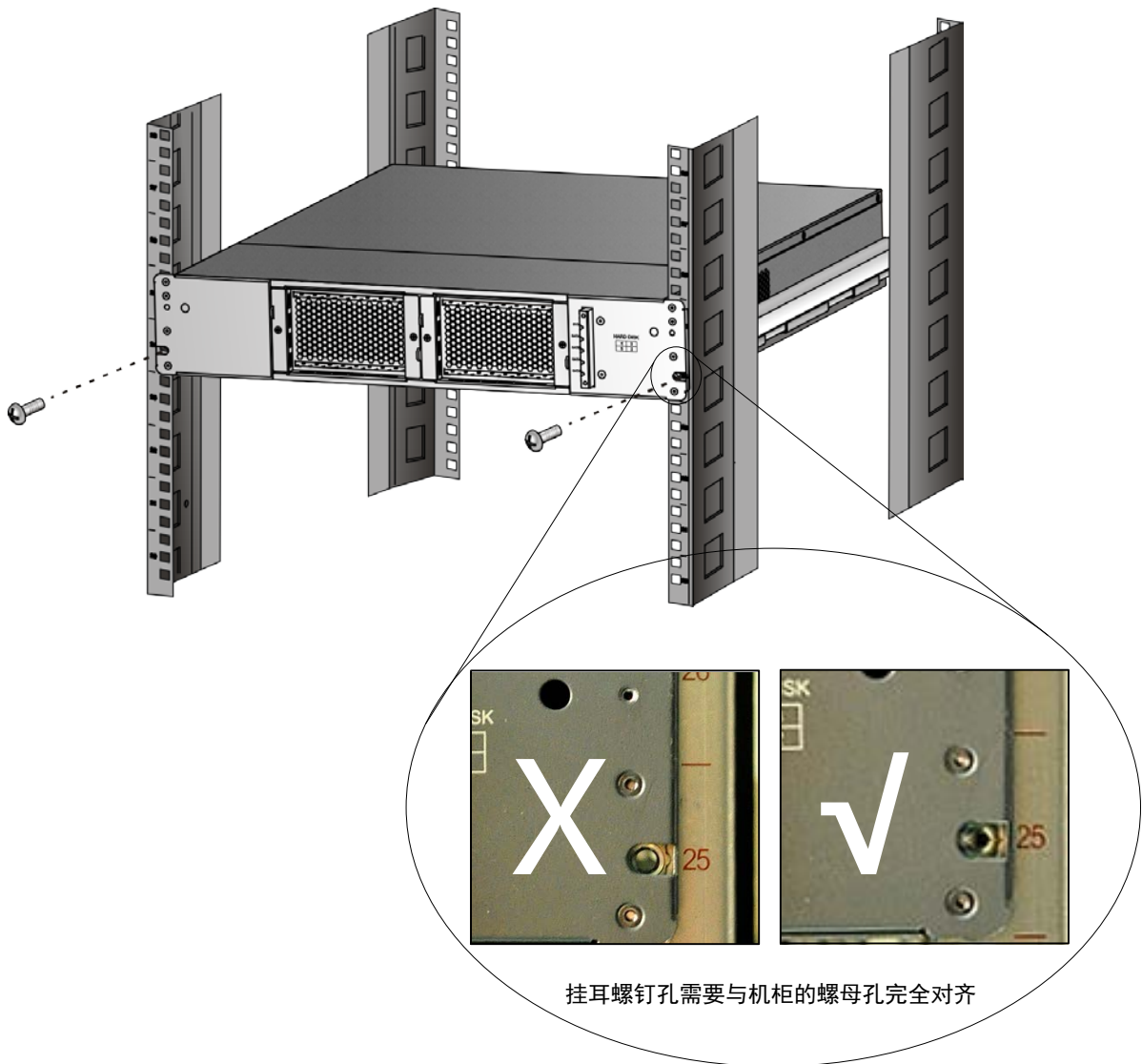
图2-5 用螺钉将挂耳固定在机柜上
