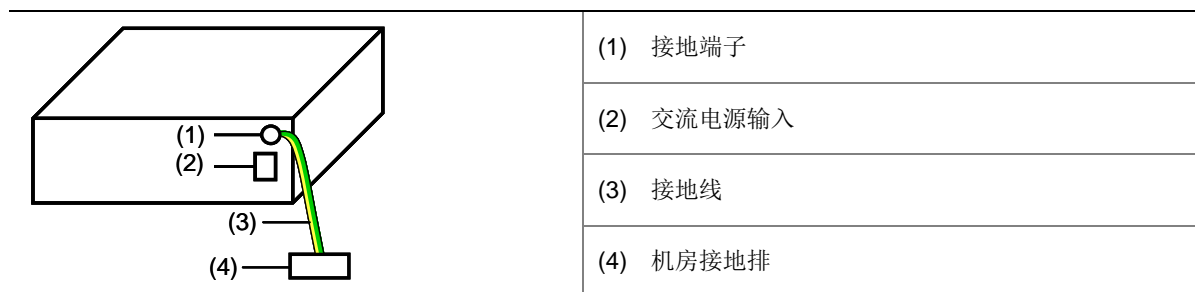
图2-12 接地安装示意图（机房有接地排）
