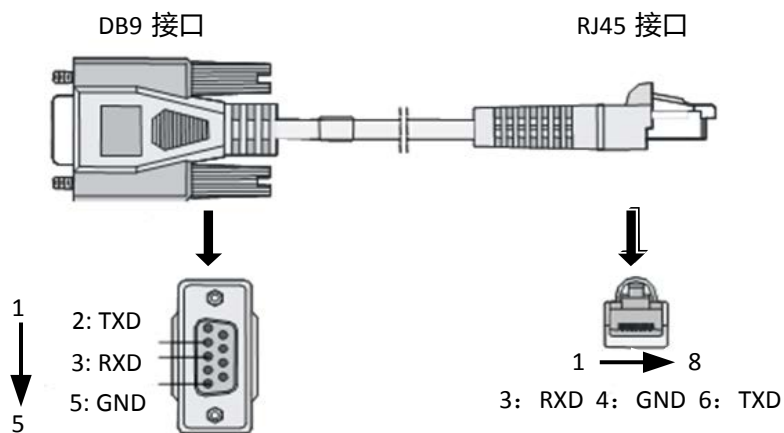
图2-11 RS232 串口线
