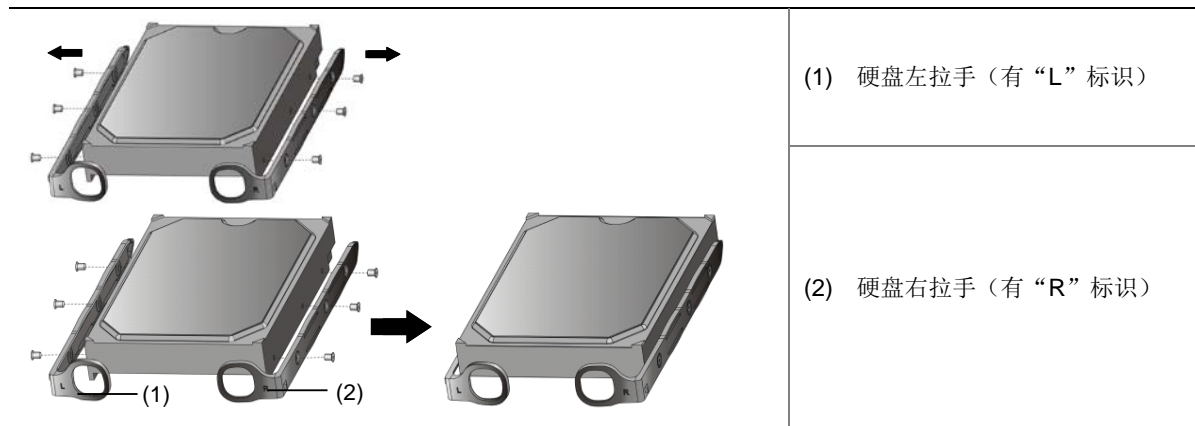
图6-2 拆卸与安装硬盘拉手条
