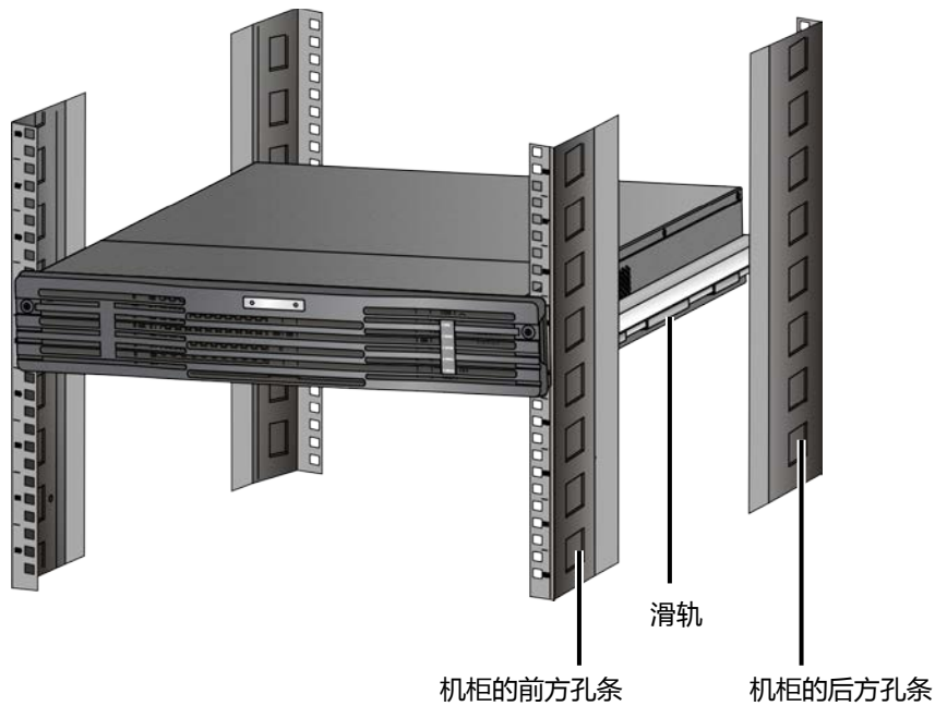
图2-3 设备安装在机柜中
