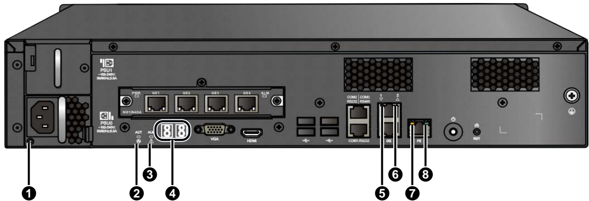
图1-5 后面板指示灯/数码管
