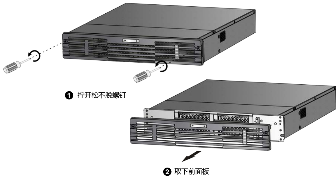
图2-2 拆卸前面板
